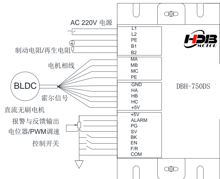
典型接线图
