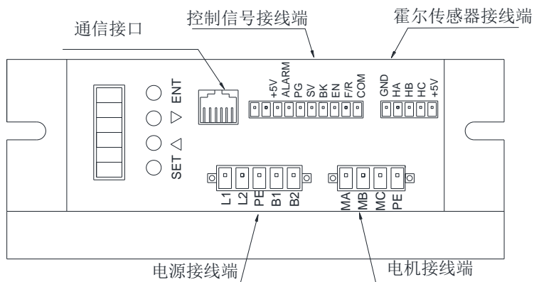
各端子在面板上的位置图
