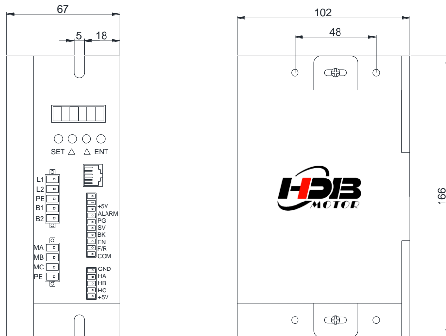
机械安装尺寸图
